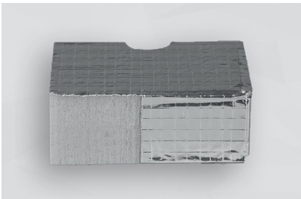
Cello® HR 290 ALG-04 afgeplakt met Cello® PLAKBAND ALU-04
